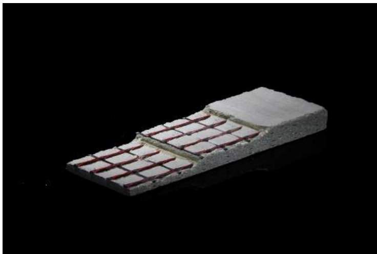
Carbontextil in Beton.jpg
